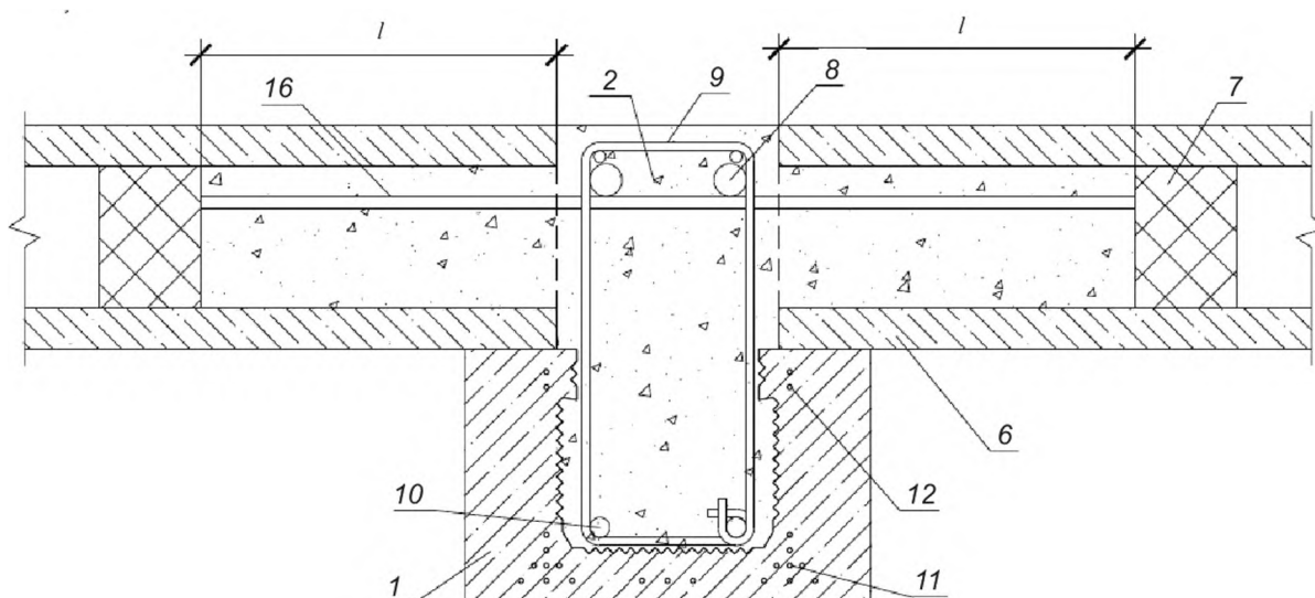
б) Узел соединения с перекрытиями
