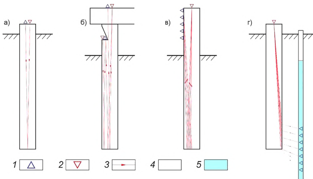
а) стандартная; б) обследование свай в составе ростверка; в) профилирование с общим пунктом возбуждения сигнала; г) обследование свай с использованием вспомогательной скважины; 1 — приемник; 2 — источник; 3 — лучевые траектории распространения упругих волн; 4 — железобетон; 5 — заполненная водой скважина
